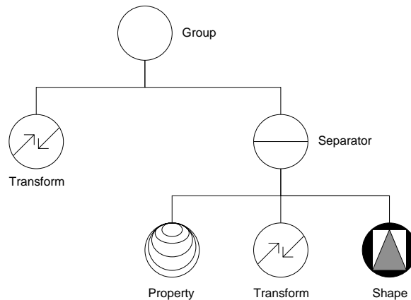
Figura 8: Exemplo de grafo de cena.
